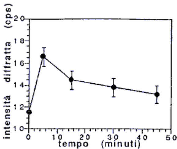
Figura 5 Risposte diffrattometriche del crisotilo in funzione del tempo di macinazione. I dati si riferiscono a campioni di 400 µg di amianto-cemento
